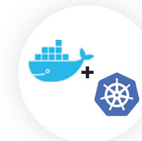
Docker & Kubernetes
